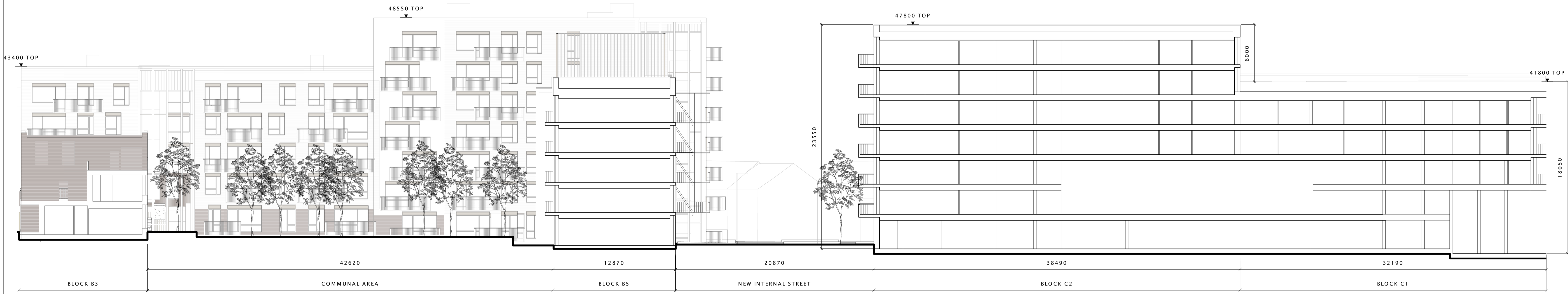
2 SITE LONG SECTION 2/3 1 : 200
